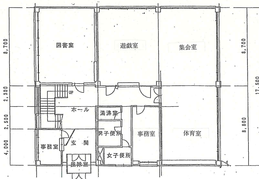
1階平面図 S=1/300
