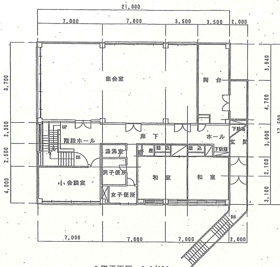
2階平面図 S=1/300
