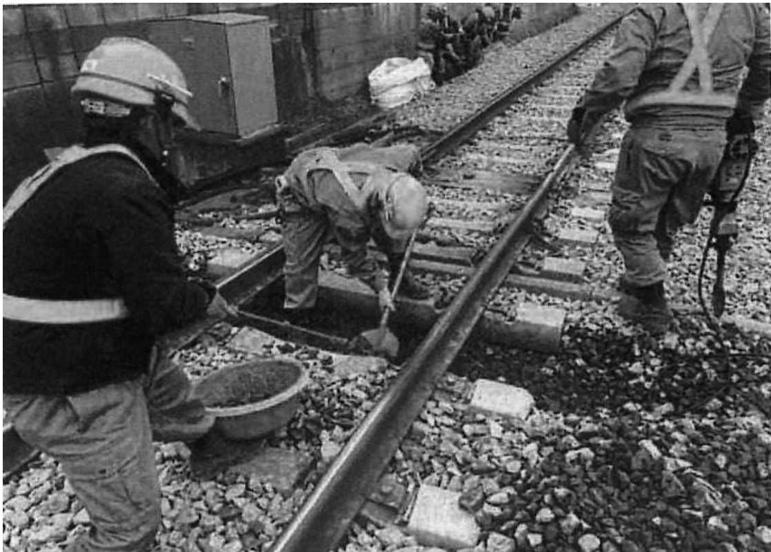
軌道修繕工事（緒ヶ崎駅～平和台駅間）
