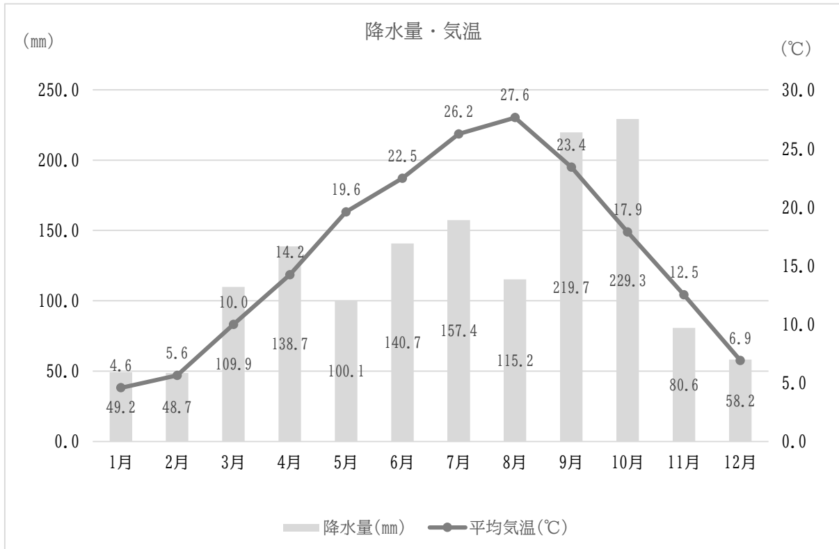
図 1-5-5 過去 10 年間の平均降水量と平均気温の分布（平成 25 年～令和 4 年）
