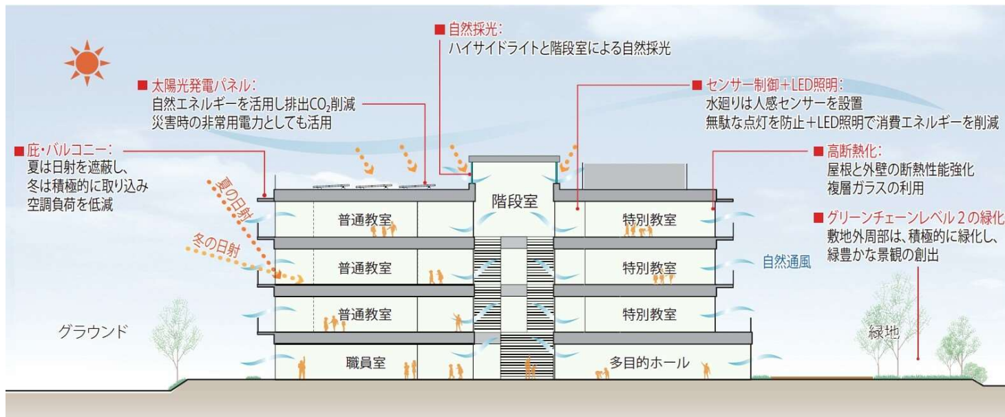
パッシブメインなエコスクールイメージ(断面図)
