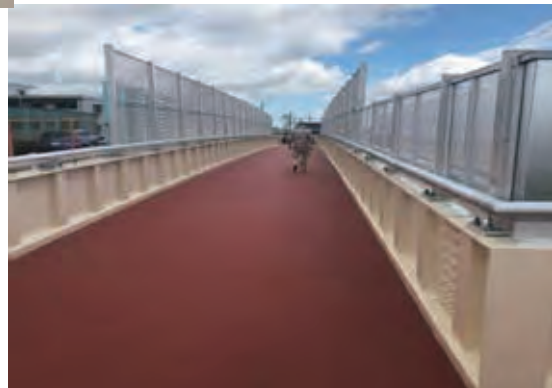
新設歩道橋設置状況
