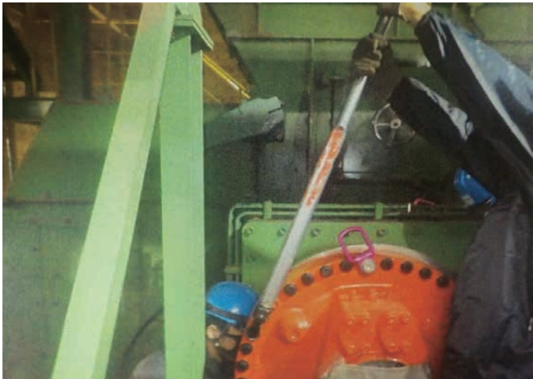
リサイクル館 粗大ごみ破碎機油圧装置整備
