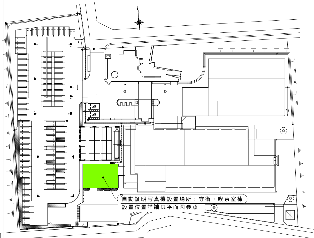
配置図：S=1/800 (A3)
