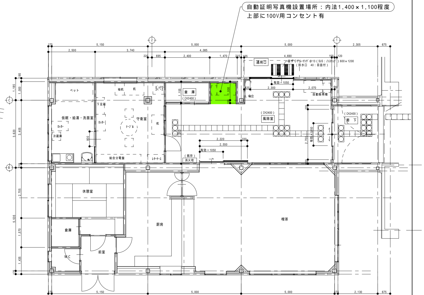
守衛・喫茶室棟平面図：S=1/100 (A3)
