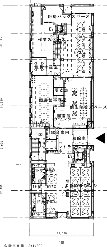
各階平面図 S=1:300
