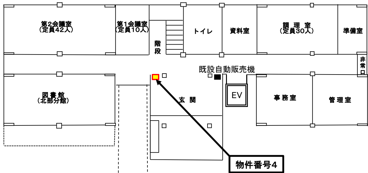
北 部 公 民 館 平 面 図
