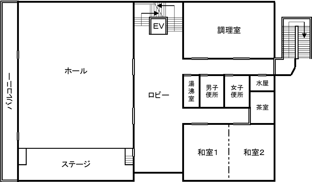
2階平面図
