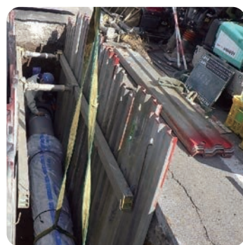
▲配水管を吊り下げて設置している様子
