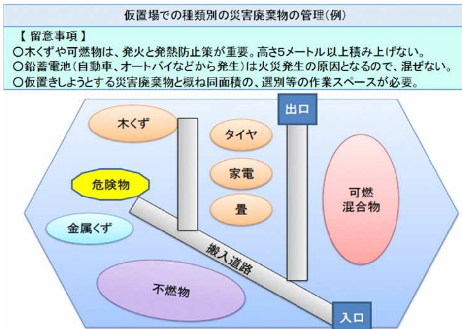
図3-10 仮置場のレイアウトイメージ
