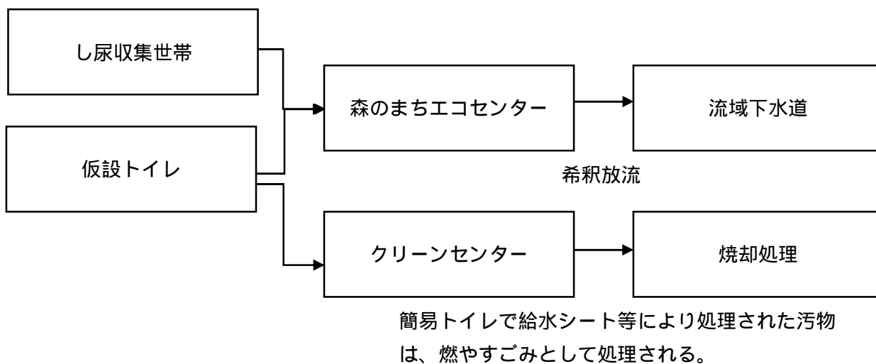
図2-4 し尿の処理フロー
