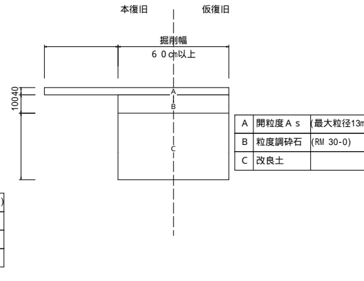
D - 1 歩道(乗入部)
