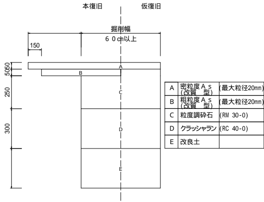
A - 1 幹線・補助幹線道路 (幅員：1.6m以上)
