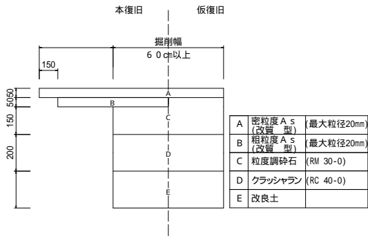
A - 2 幹線・補助幹線道路 (幅員：1.6m未満)
