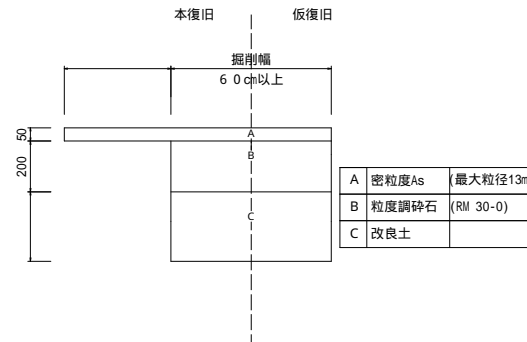
D - 2 歩道(乗入部) (準中型車以上又は通行車両が多い場合)
