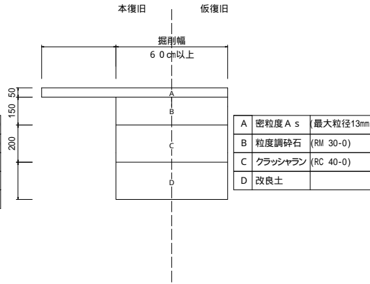
B - 1 区画道路 (幅員：4.5m以上)
