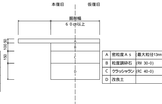
B - 2 区画道路 (幅員：4.5m未満)
