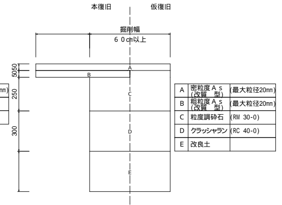
D - 3 歩道(乗入部) (大型車)
