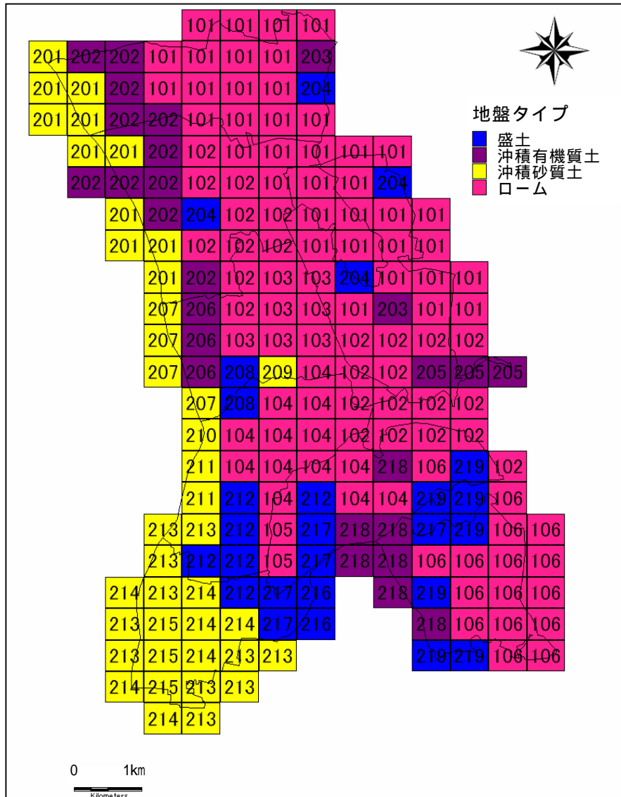
図 地盤モデル図
