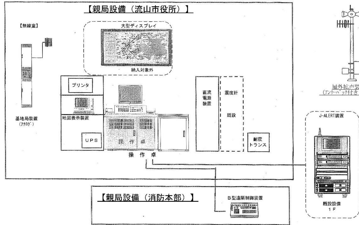
図 3-2-5 市防災行政無線固定系系統図
