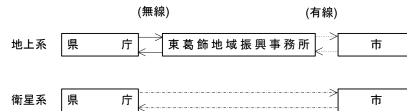
図 3-2-7 県との通信経路
