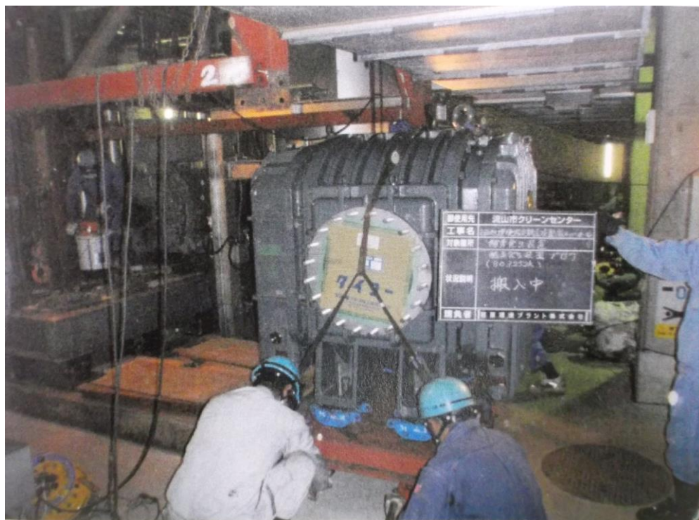
酸素発生装置ブロー整備中の様子
