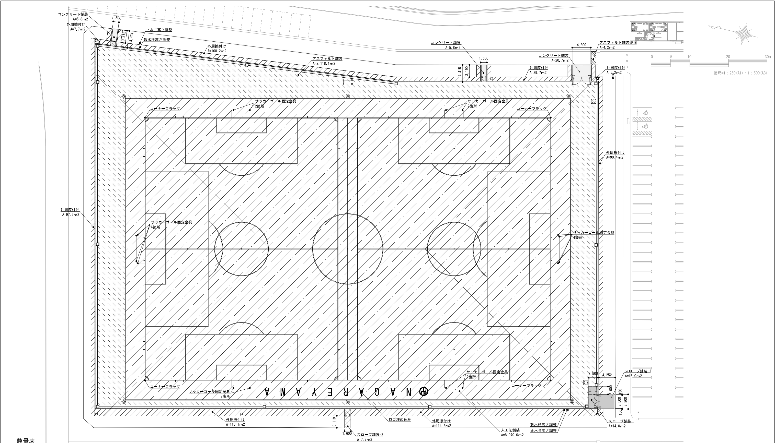
舗装・施設計画平面図 S=1:250
