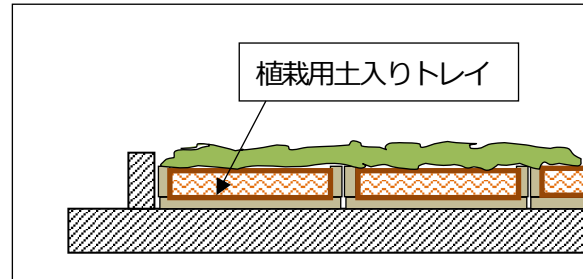
床面上に、軽量土等の植栽基盤を有したトレイ を設置し、地被植物等を植栽する例
