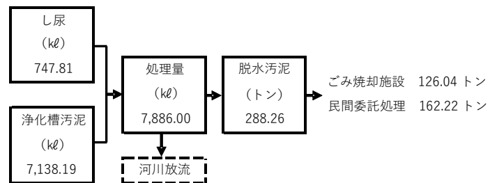
し尿処理フロー
