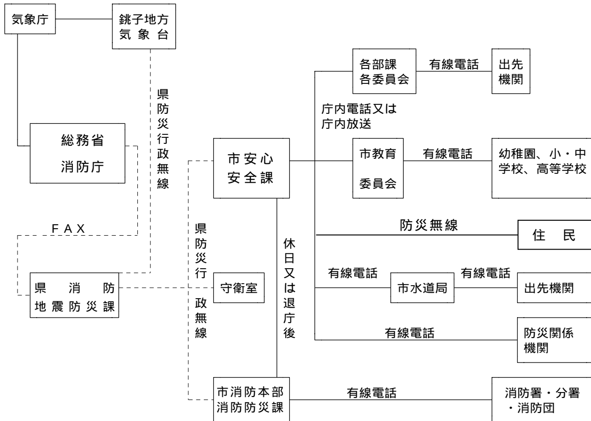
図 東海地震注意情報の伝達系統・伝達手段
