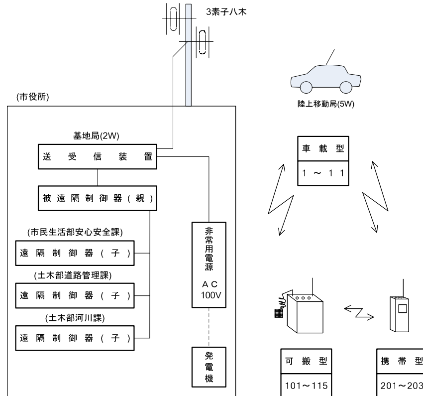
図 市防災行政無線移動系系統図
