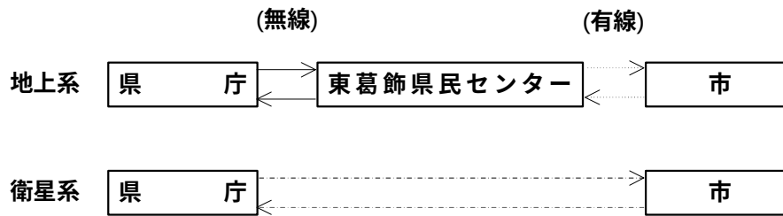
図 県との通信経路
