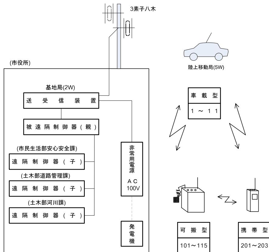
図 市防災行政無線移動系系統図
