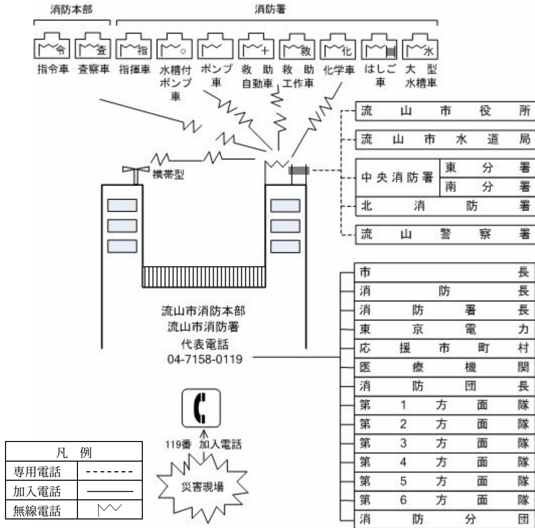
図 消防通信系統図
