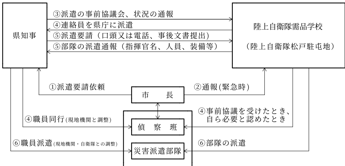
図 自衛隊災害派遣要請系統図
