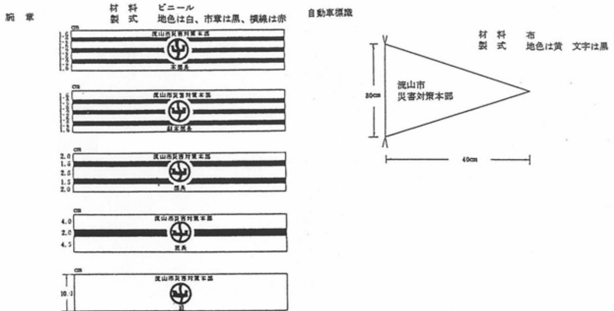
図 腕章及び自動車標識
