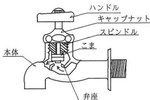
図VI-2-1 一般的な給水栓の構造
