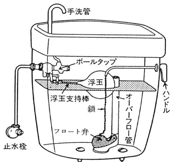
図-VI-2-2 トイレロータンの構造
