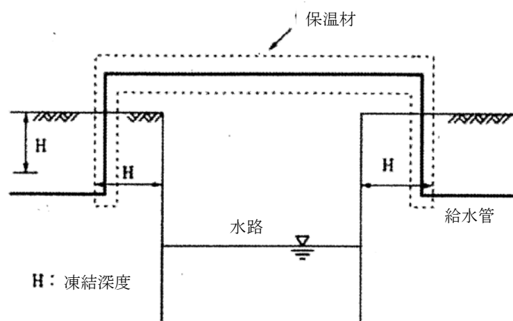
図Ⅱ-13-30 水路横断間の防寒措置
