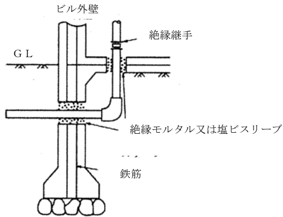
図Ⅱ-13-17 ビルに入る配管の絶縁概要図
