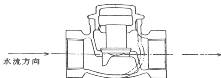
図Ⅱ-13-25 リフト逆止弁
