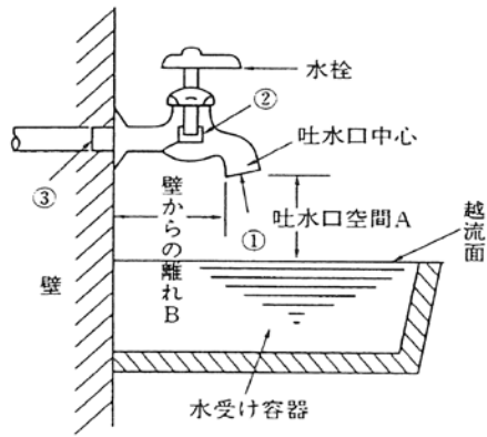
図 II-13-18 洗面器等の場合
