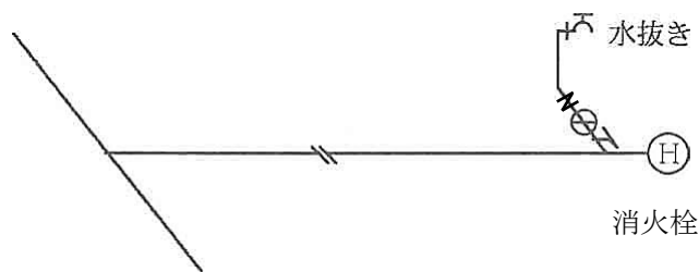
図Ⅱ-12-1 私設消火栓設置例
