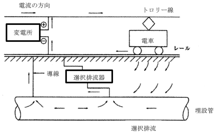
図Ⅱ-13-16 選択排流法
