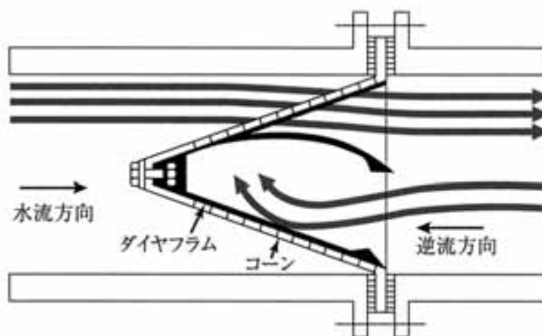
図Ⅱ-11-27 ダイヤフラム式
