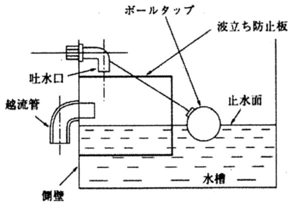
図Ⅱ-13-2 受水槽の波立ち防止板
