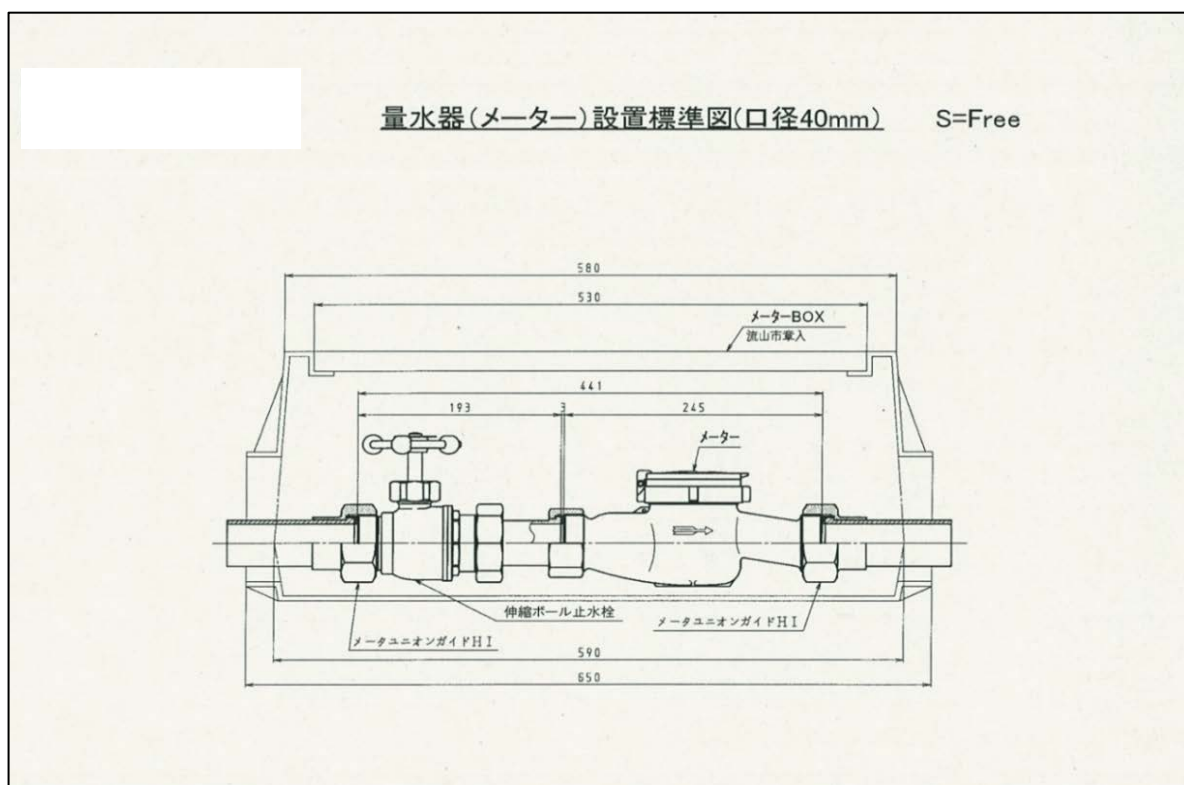
図Ⅱ-11-2 メーターボックス構造例 (40mm)
