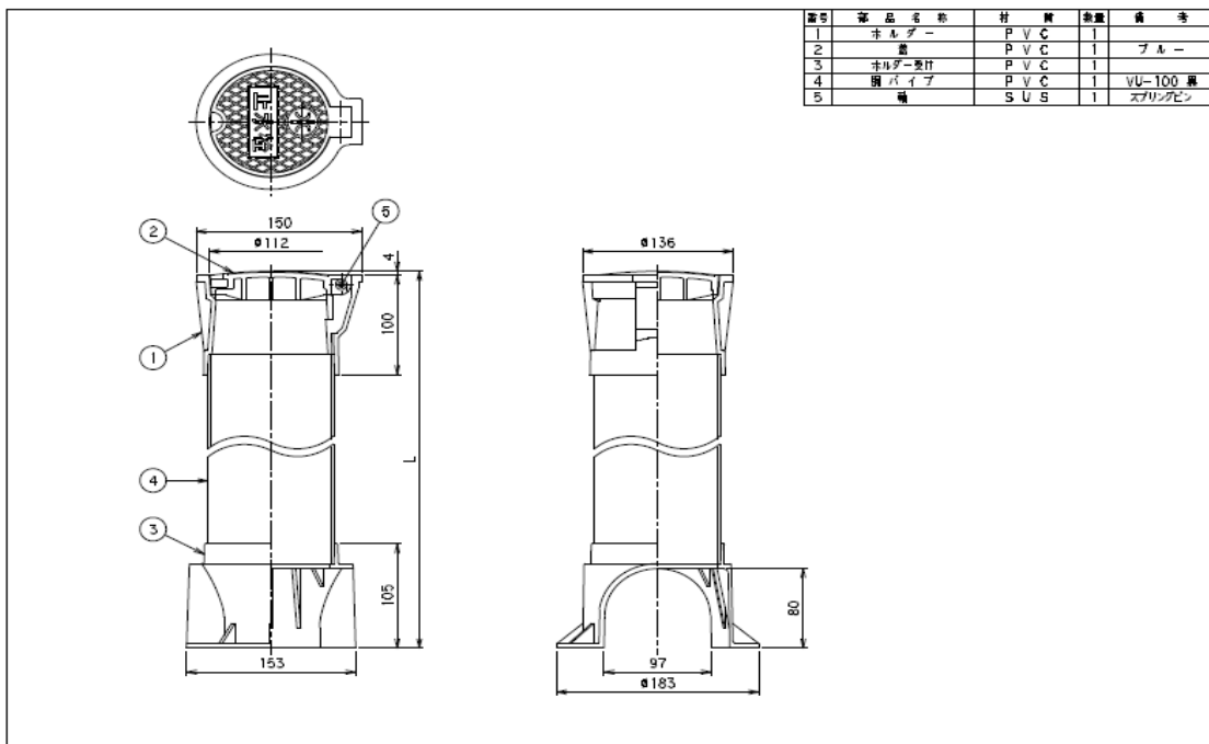
図 II-10-2 樹脂製止水栓篋100型
