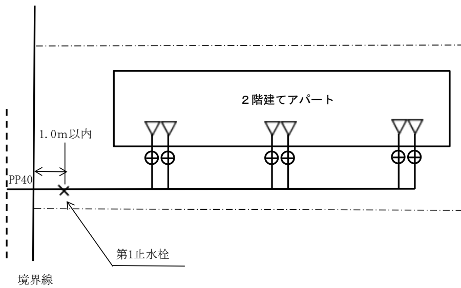
II-10-6 設置標準図 (連合給水装置 アパート等)
