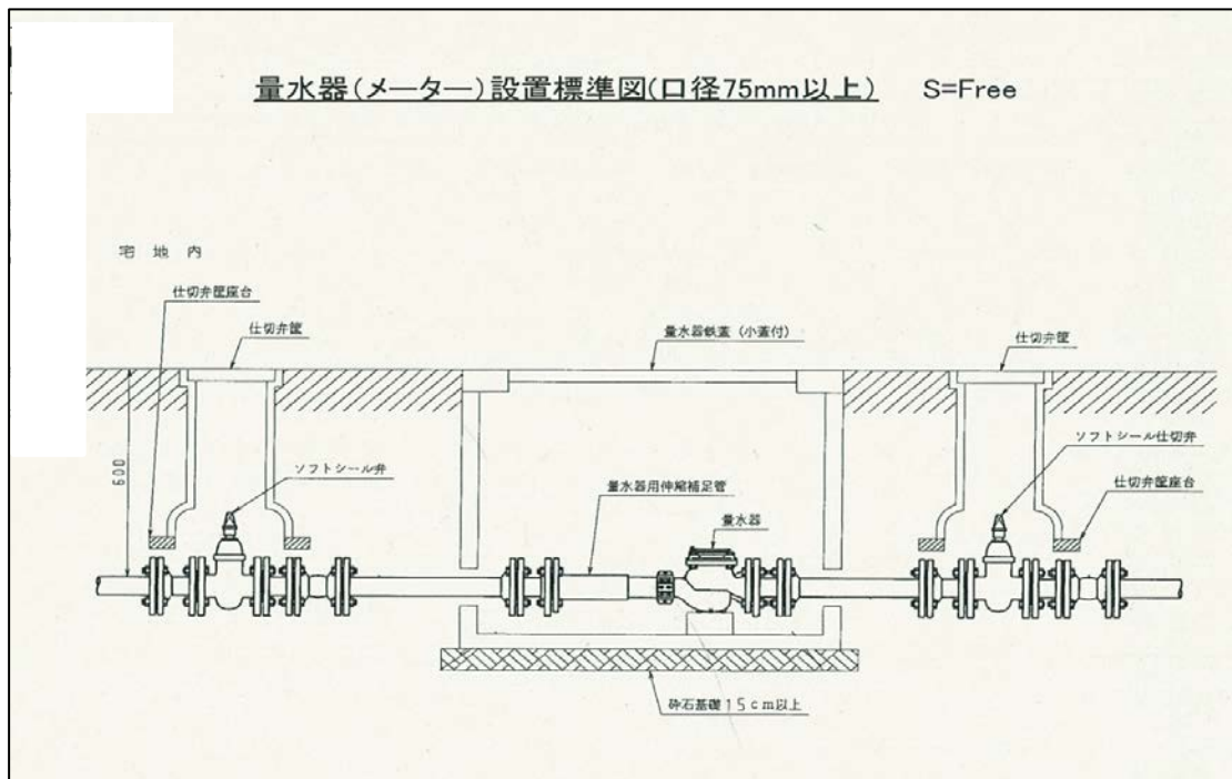
図II-11-4 メーターボックス構造例 (75mm)
