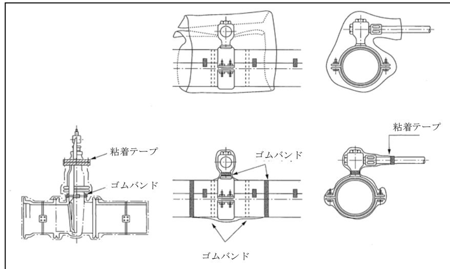
図Ⅱ-13-11 サドル付分水栓等外面防食
