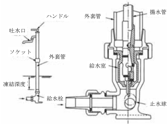
図II-13-31 内部貯留式不凍給水栓
