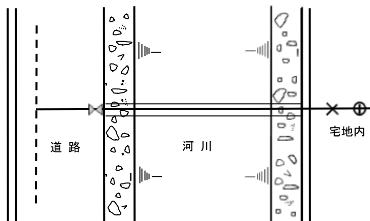
II-10-8 設置標準図 (水路横断)
