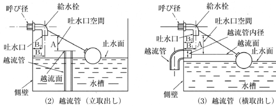
図 II-13-18 洗面器等の場合
