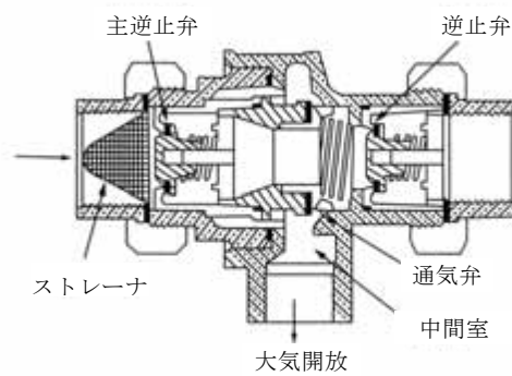
図Ⅱ-13-23 中間室大気開放式逆流防止器
