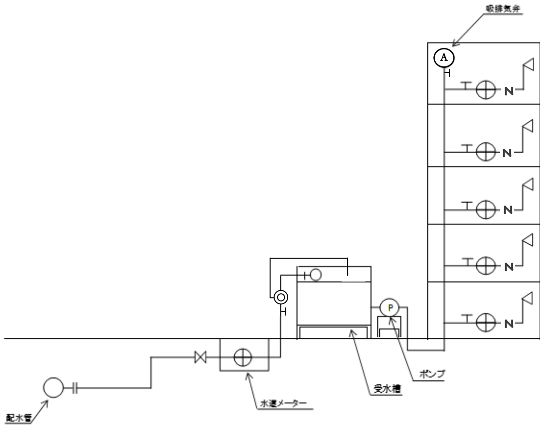
図 II-7-1 受水槽方式（ポンプ直送式）の形態
