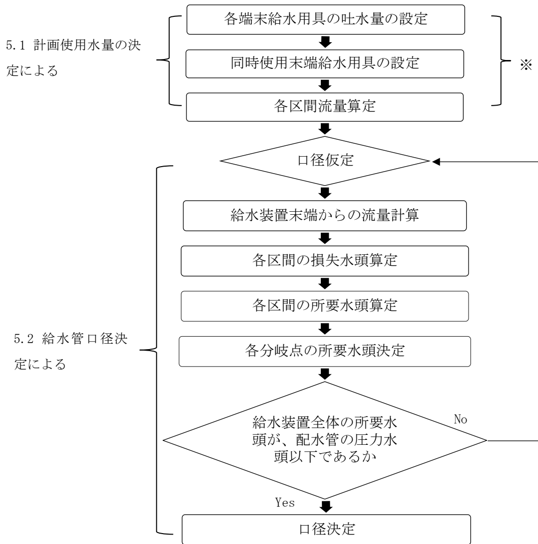
図Ⅱ-5-3 口径決定の手順
