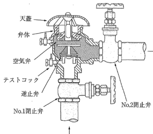
図Ⅱ-13-28 圧力式
