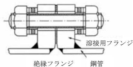
図Ⅱ-13-15 電氣的絶縁継手
