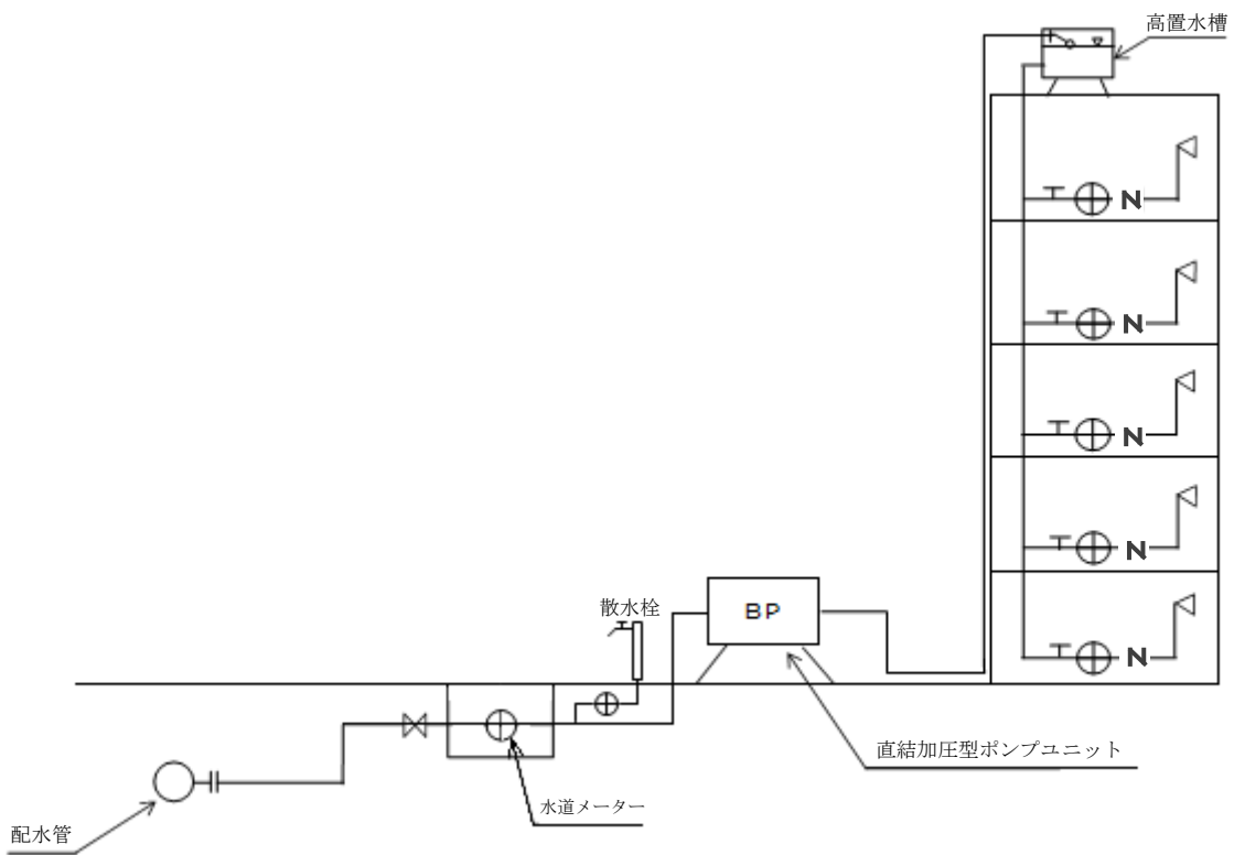
図 II-6-2 直結増圧式（ポンプ直送式）の形態
