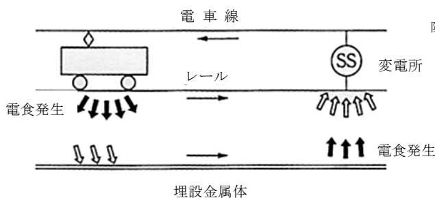
図 II-13-5 漏えい電流による電食
