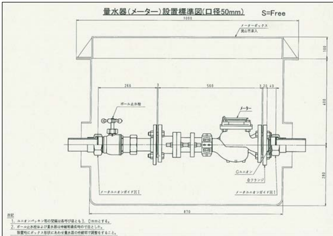
図II-11-3 メーターボックス構造例 (50mm)
