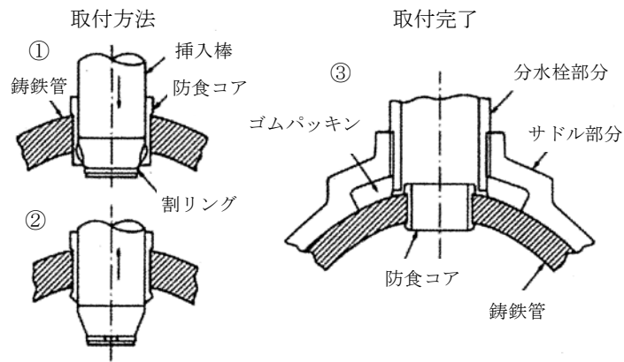
図Ⅱ-13-13 管の内面の防食
