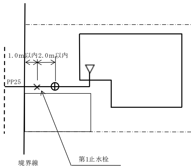
図Ⅱ-10-4 設置標準図（一般家屋）
