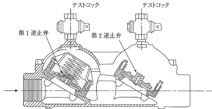
図Ⅱ-13-22 二重式逆流防止器
