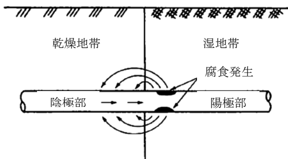
図Ⅱ-13-9 通気差による浸食
