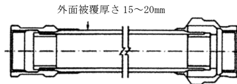
図Ⅱ-13-14 電氣的絶縁物による管の被覆
