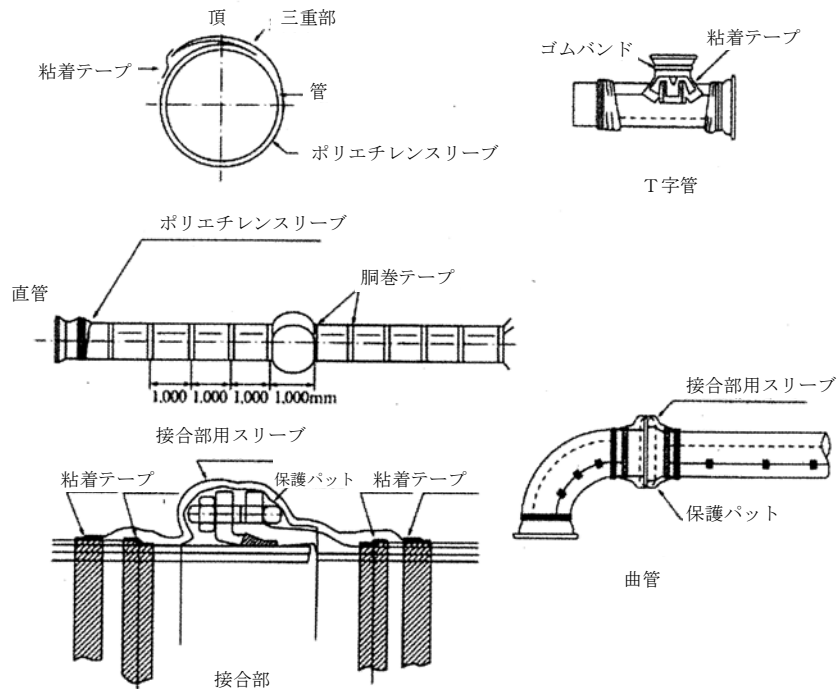
図 II-13-12 ポリエチレンスリーブによる被覆
