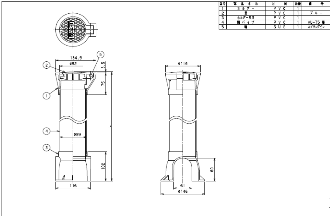
図 II-10-1 樹脂製止水栓篋75型
