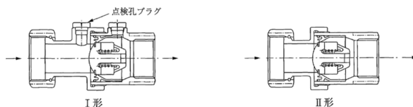
図Ⅱ-13-20 単式逆流防止弁
