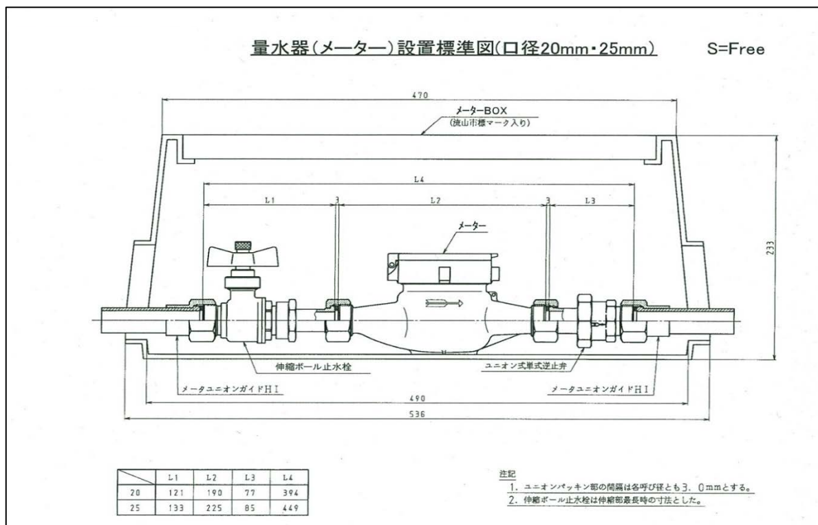
図Ⅱ-11-1 メーターボックス構造例 (20mm・25mm)
