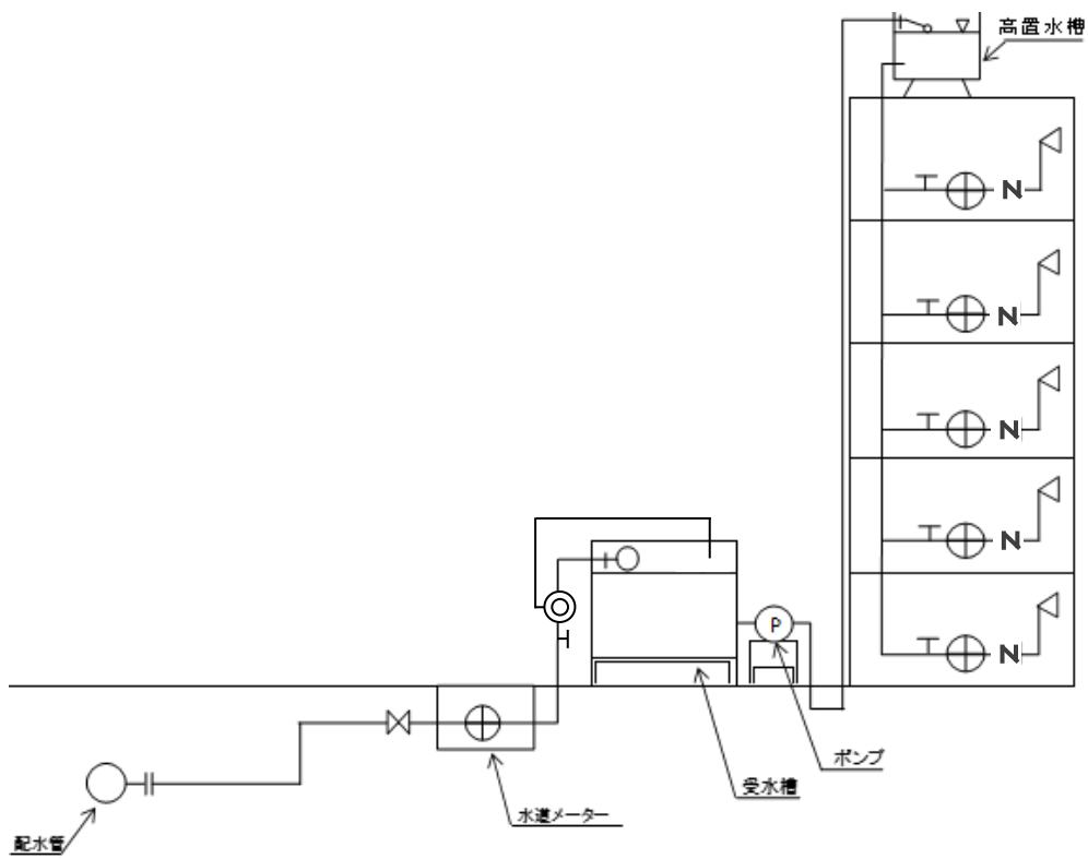
図 II-7-2 受水槽方式（高置水槽式）の形態
