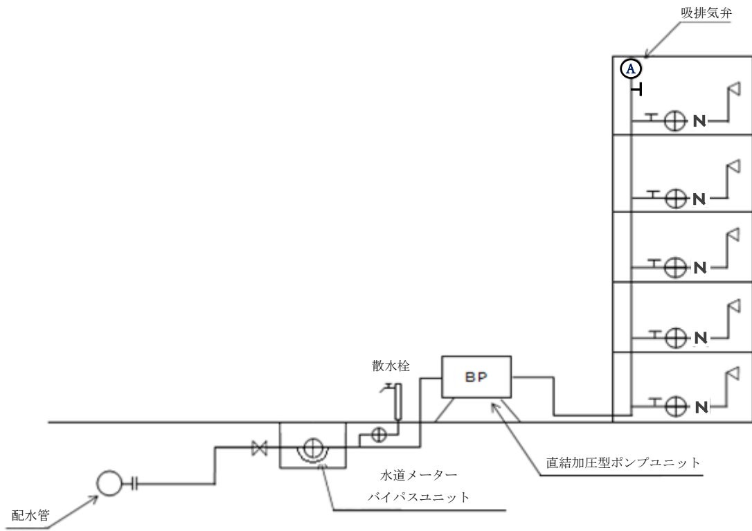
図 II-6-2 直結増圧式（ポンプ直送式）の形態
