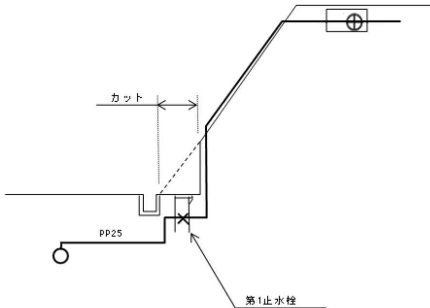
II-10-7 設置標準図 (法面配管)
