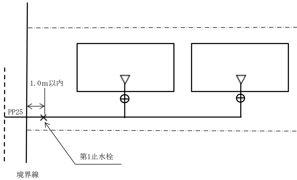
II-10-5 設置標準図 (連合給水装置)
