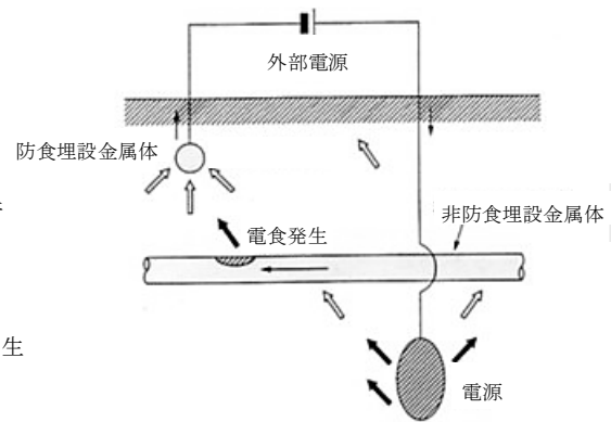
図 II-13-6 干渉による電食
