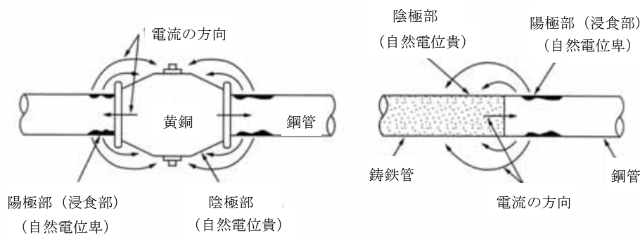
図Ⅱ-13-7 異種金属接触による侵食
