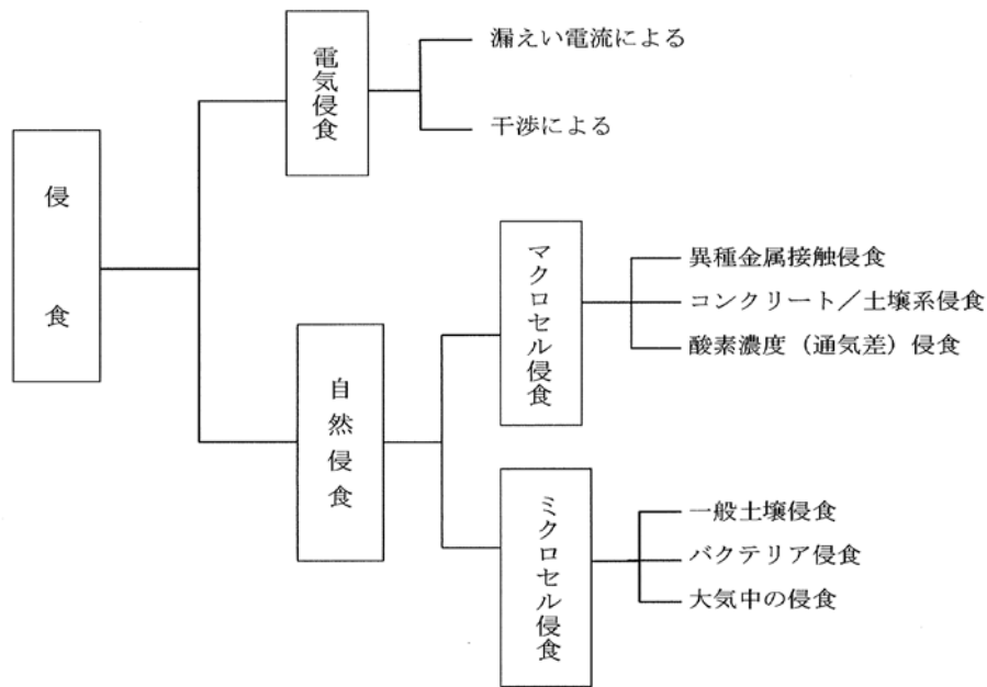
図 II-13-4 侵食の種類
