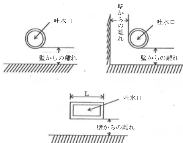
図 II-13-19 水槽等の場合 (2)
