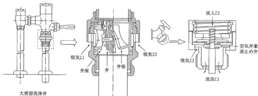
図Ⅱ-13-29 大気圧式
