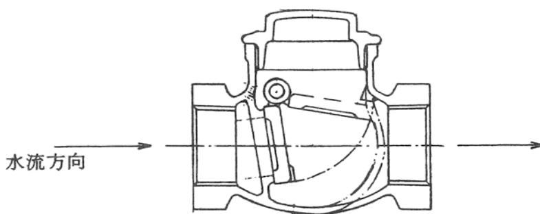
図Ⅱ-13-26 スイング逆止弁
