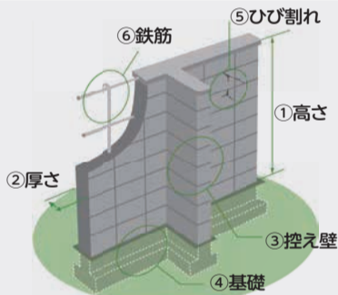
出典：パンフレット「地震からわが家を守る」日本建築防災協会2013.1より一部改
