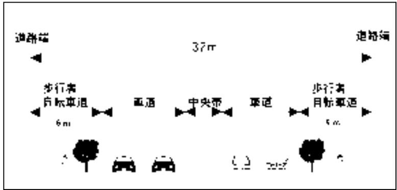
道路の断面図
