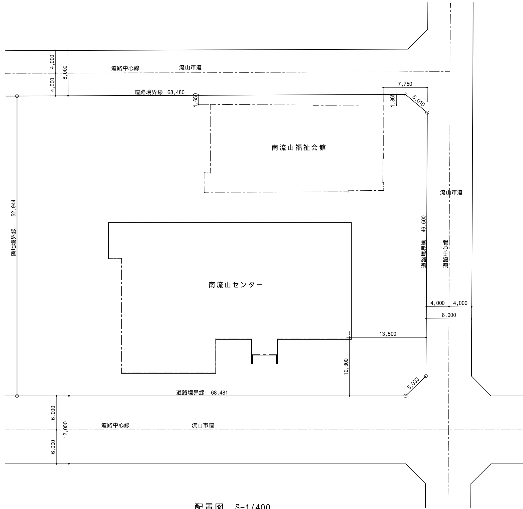
配置図 S=1/400
