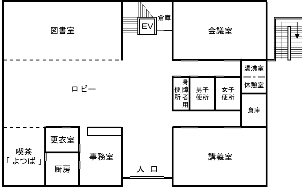
1階平面図
