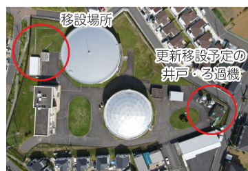
西平井浄水場全体図
