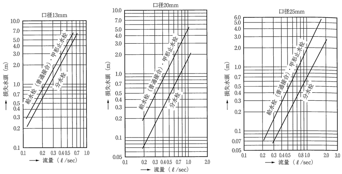
図VII-2-6 水栓類の損失水頭
