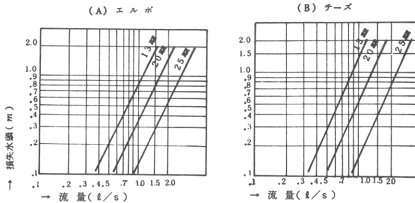
図VII-2-8 管継手類による損失水頭
