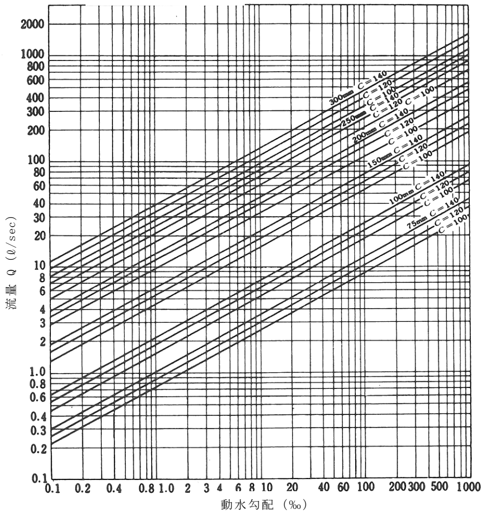
図VII-2-3 ヘーゼン・ウィリアムス公式の流量図
