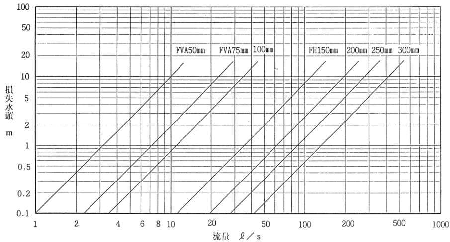
図VII-2-7 メーターの損失水頭
