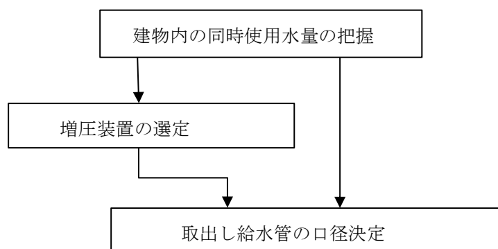
図VII-2-21 直結増圧式給水における口径決定の手順
