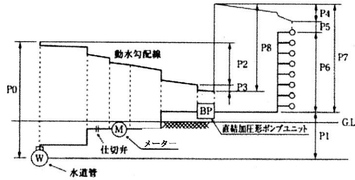
図VII-2-22 直結増圧式給水における動水勾配図
