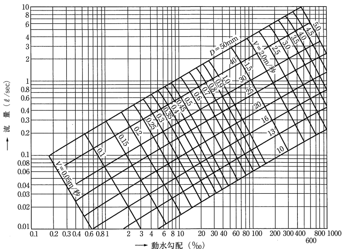
図VII-2-2 ウェストン公式の流量図
